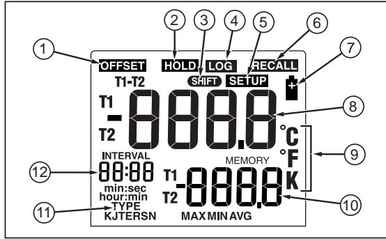
그림 2. 디스플레이 구성요소
