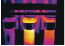
퓨즈 과열
