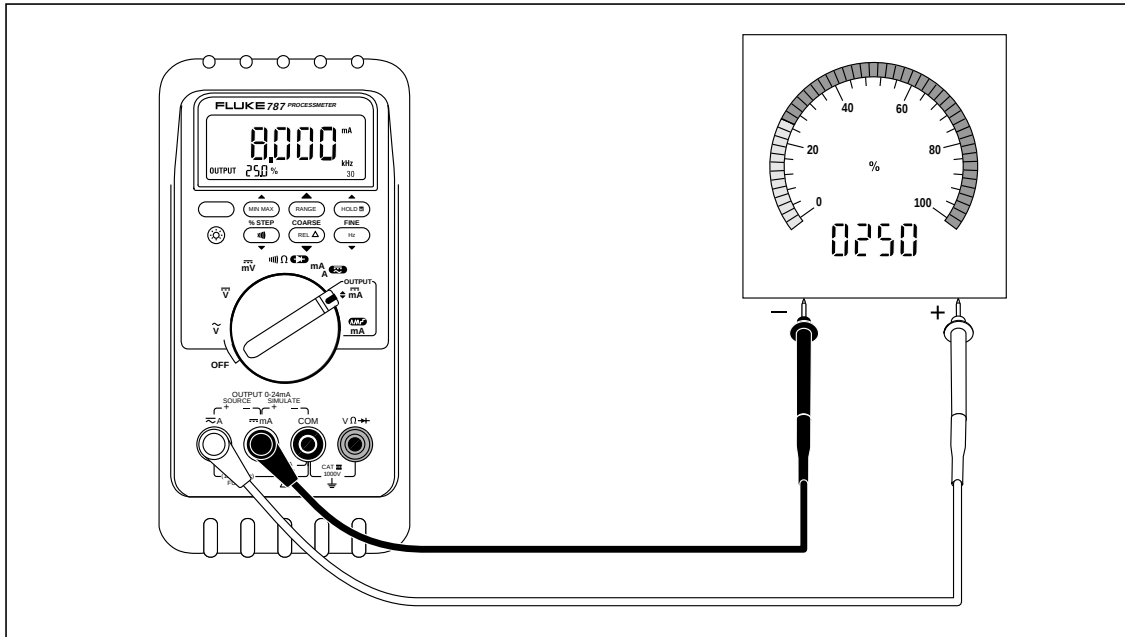
그림 7. 전류 공급
