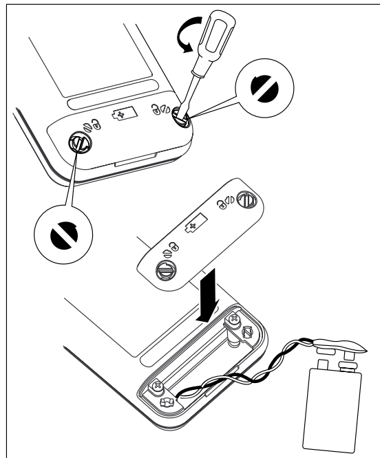
그림 10. 배터리 교체
