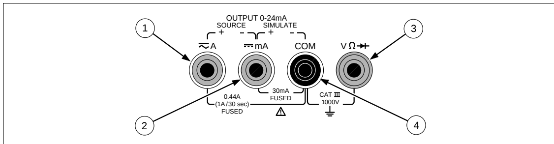
그림 2. 입력/출력 잭
