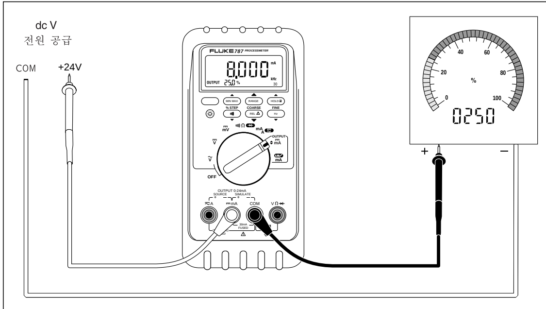
그림 8. 트랜스미터의 시뮬레이팅
