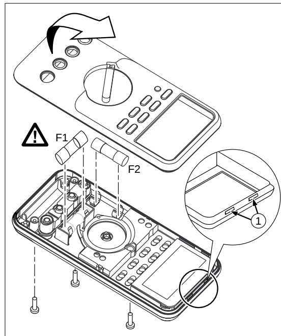
그림 11. 퓨즈 교체
